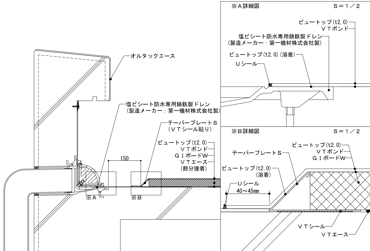
接着断熱工法 横引きドレン廻り(新築)
