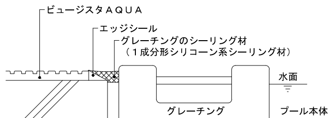
取りあい部分（グレーチング）
