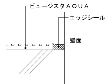
取りあい部分（壁面の端部）
