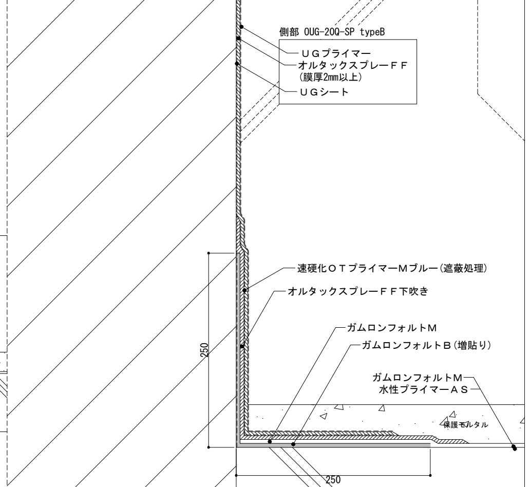
底部・側部取り合い詳細 (A3 s=1/5)
