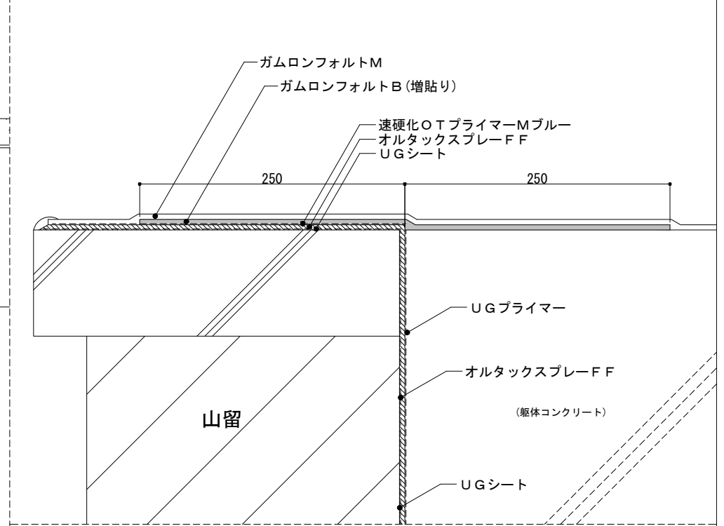
底部・側部取り合い詳細 (A3 s=1/5)
