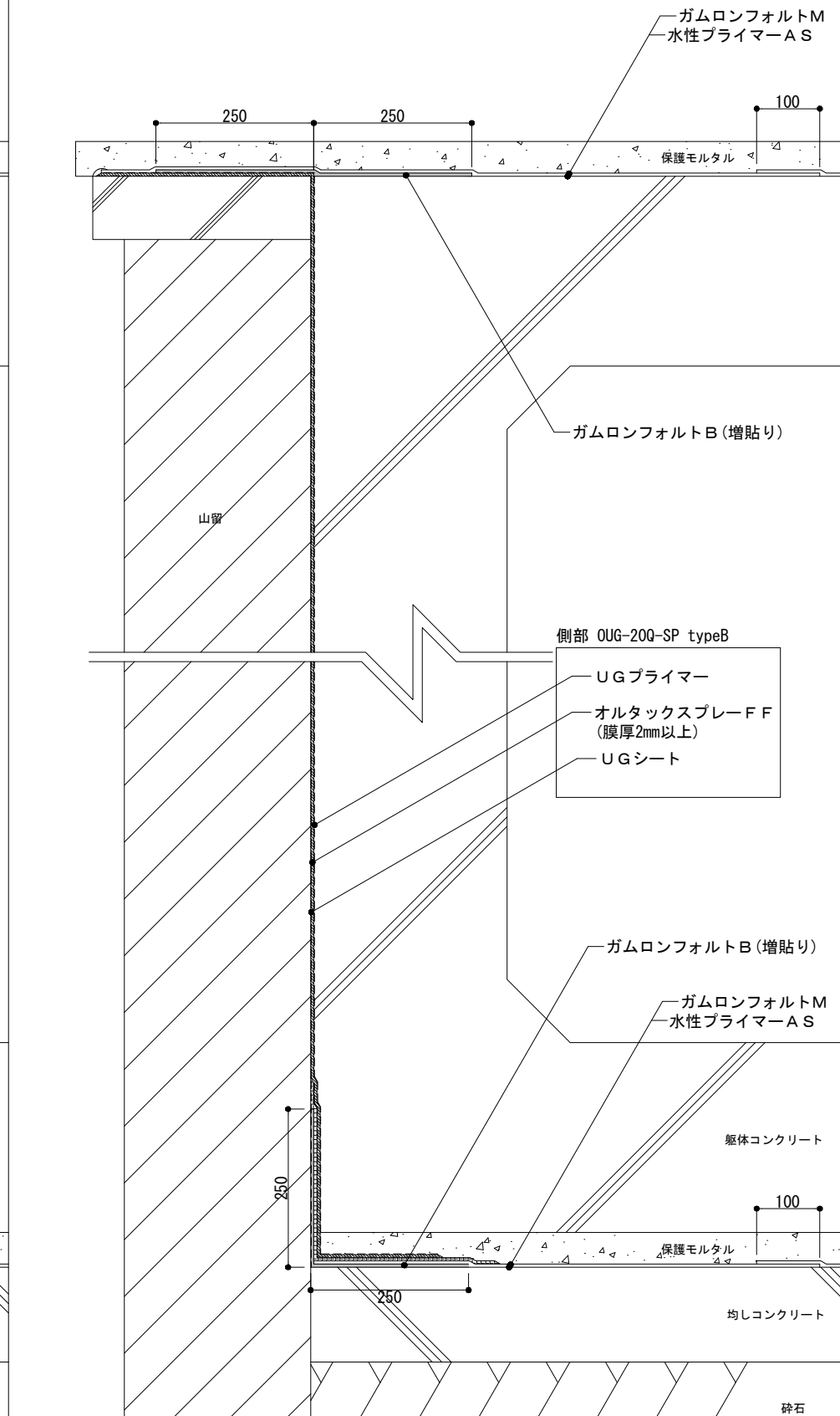
底部・側部取り合い詳細 (A3 s=1/5)
