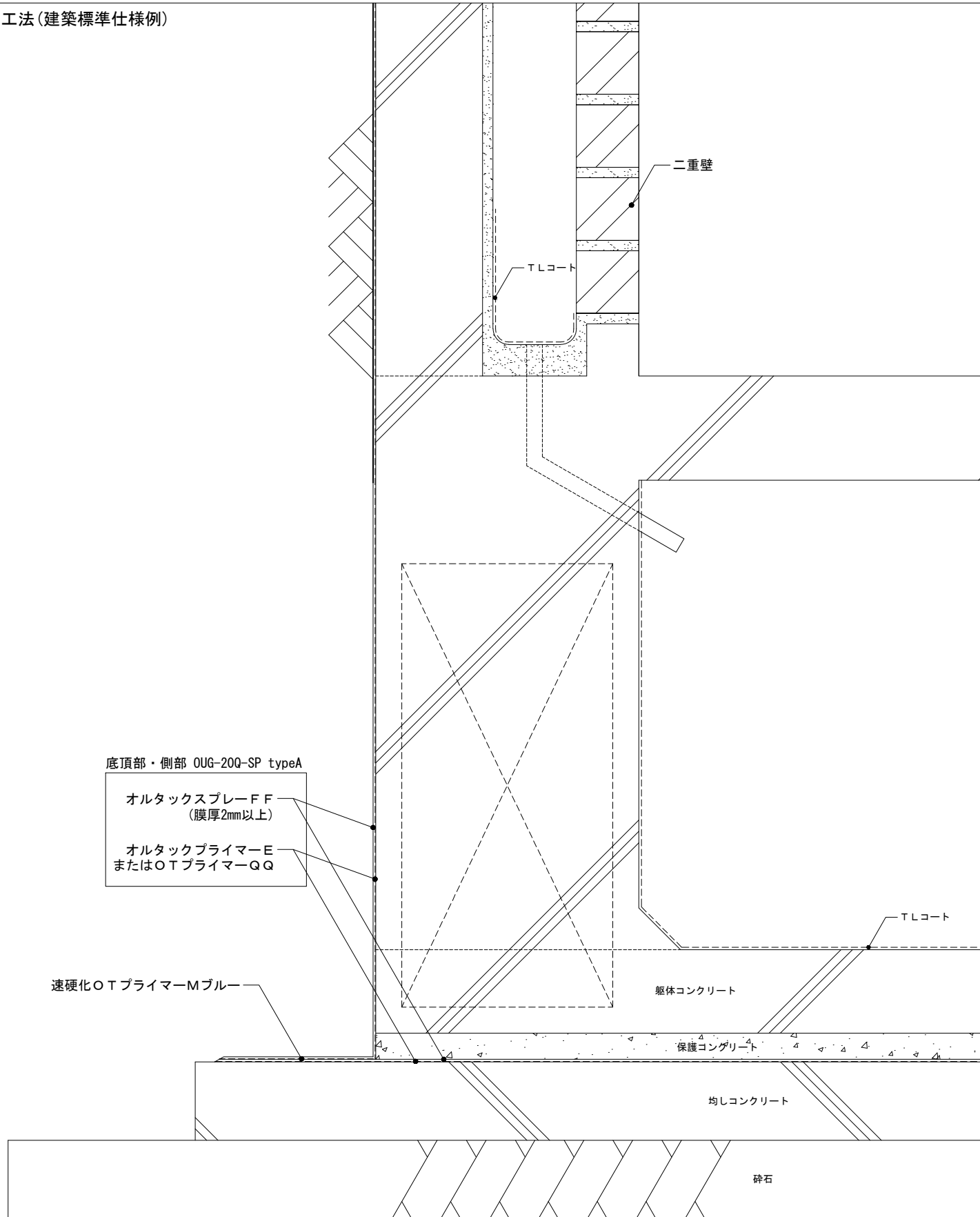
先やり工法(土木標準仕様例)
