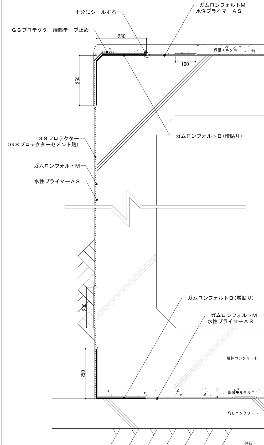
後やり工法 底部処理図 (A3 s=1/5)
