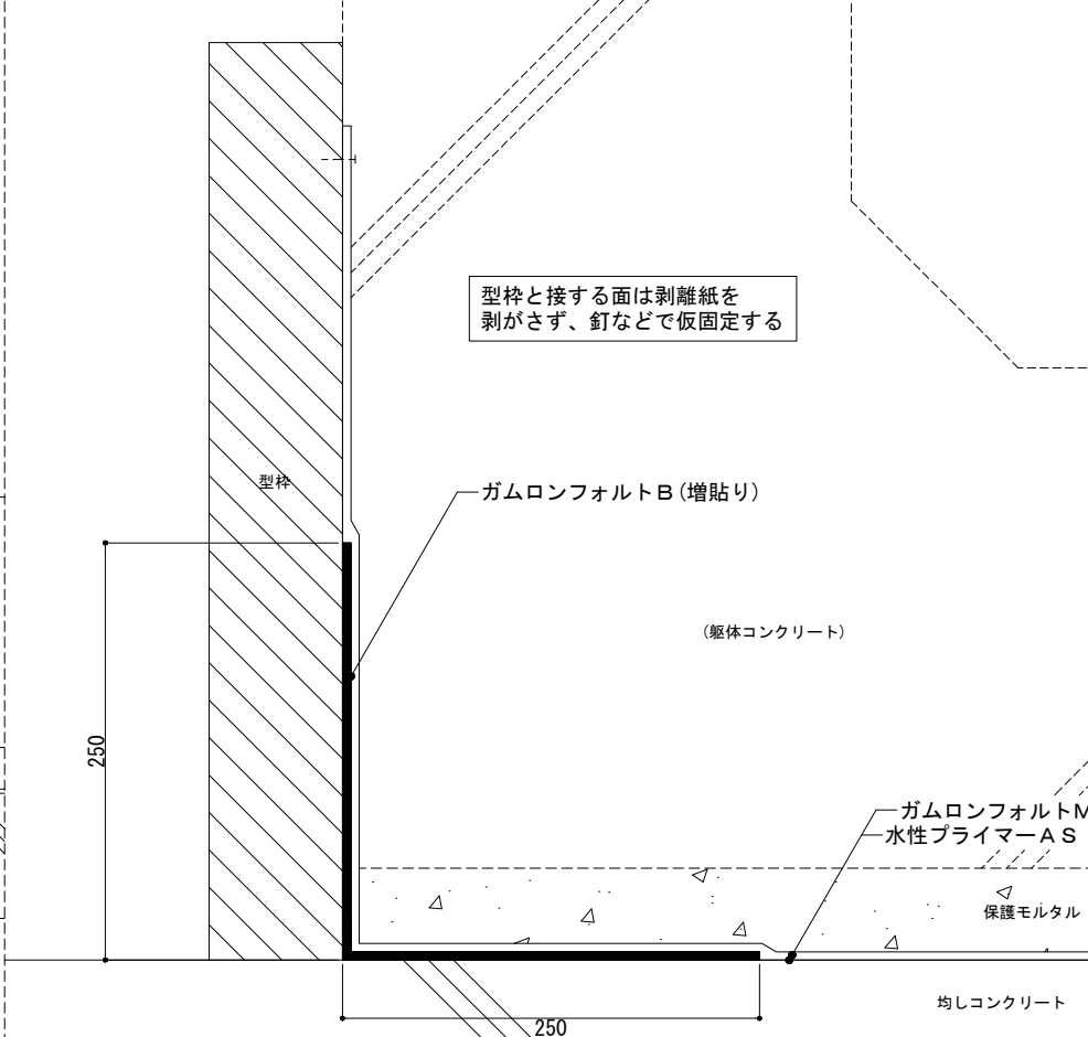
後やり工法 底部処理図 (A3 s=1/5)
