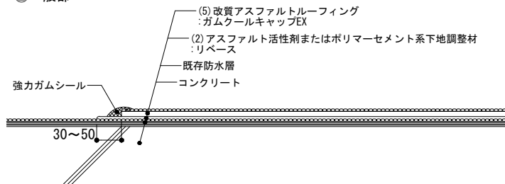
②一般部
