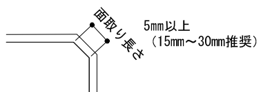
※B詳細図
