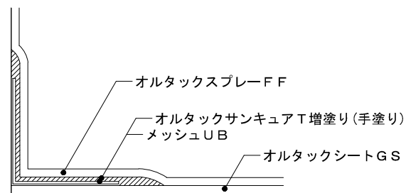
※A詳細図
