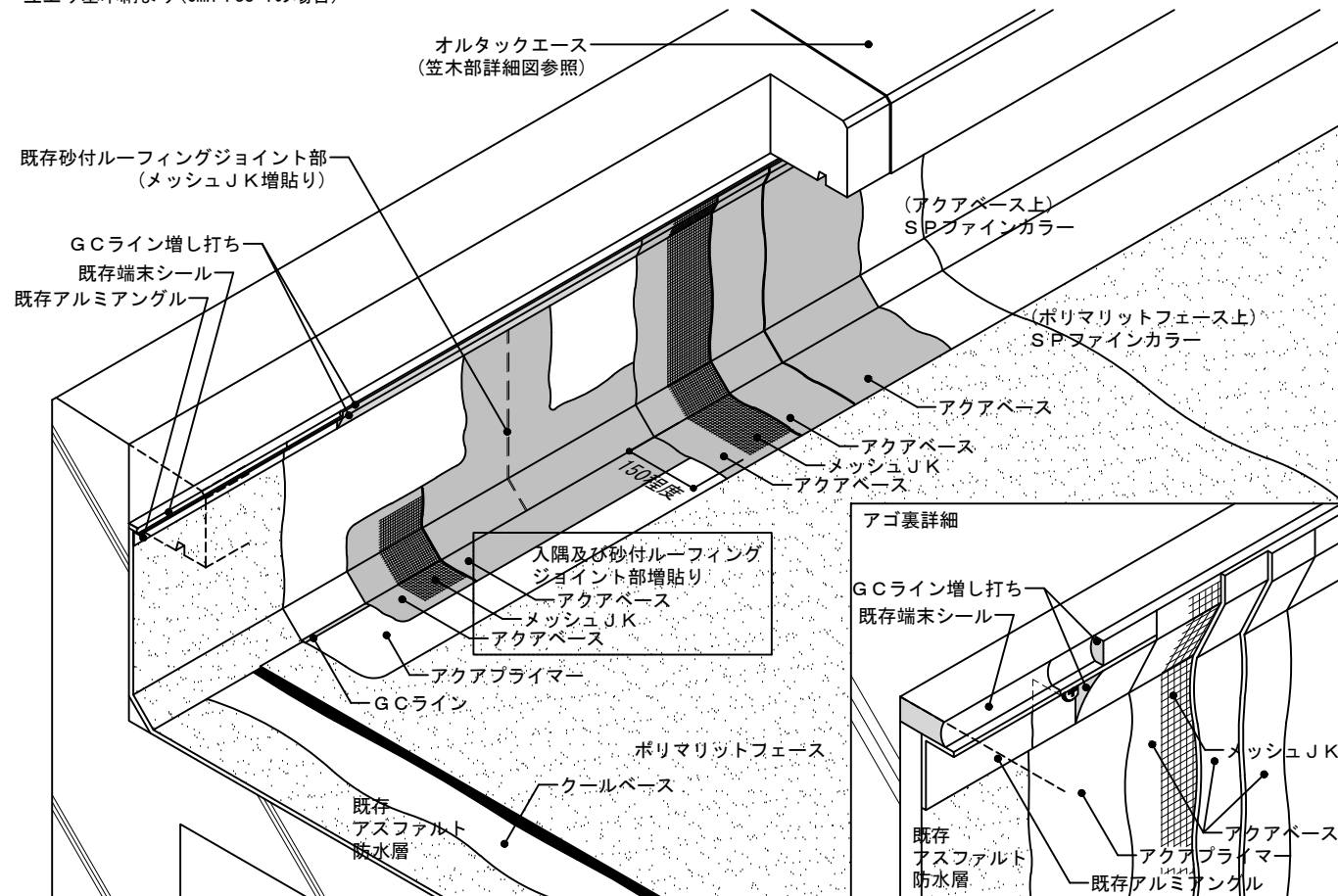
立上り基本納まり (CMH-PSS-1の場合)
